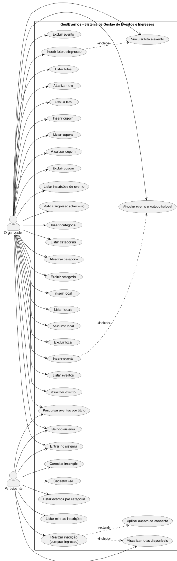
Figura 1 — Diagrama de Casos de Uso do GestEventos.
